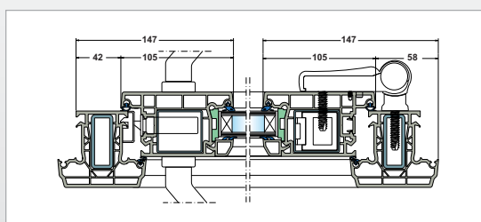
telaio Top 72 con applicazione dall'esterno
