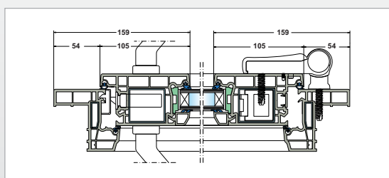
telaio da sostituzione Top 72
