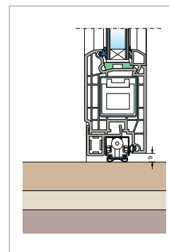
soglia codice 44 con lama parafreddo
