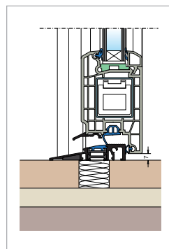
soglia codice 85 a taglio termico - profondità 72 mm
