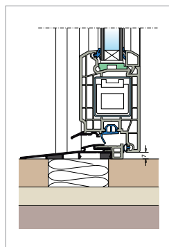
soglia codice 84 a taglio termico - profondità 110 mm
