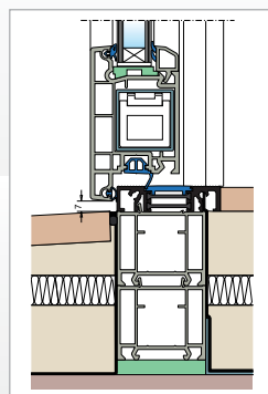
soglia codice 87A
