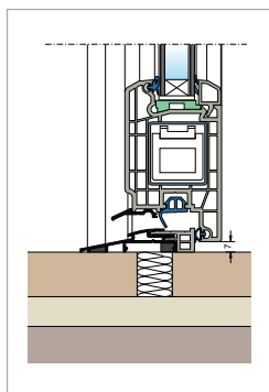
soglia codice 83 a taglio termico - profondità 77 mm
