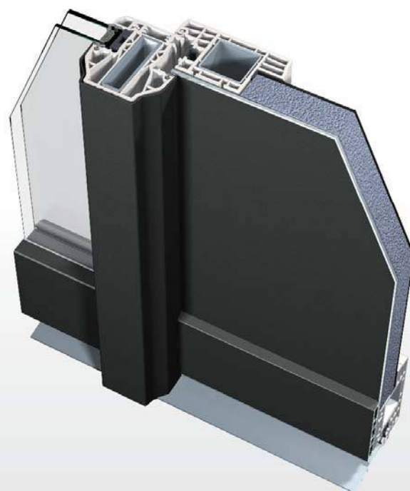
dettaglio montante fisso per portoncini con elemento laterale
