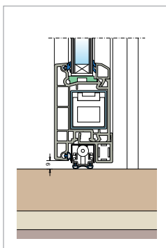
soglia codice 44A con lama parafreddo
