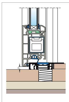
soglia codice 85A a taglio termico - profondità 88 mm
