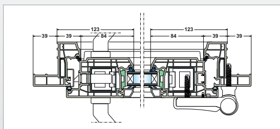
telaio da sostituzione Top 72
