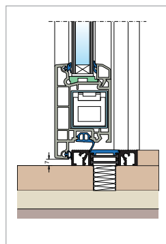
soglia codice 87A a taglio termico - profondità 70 mm
