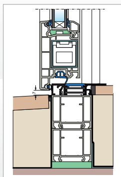
soglia codice 85A
