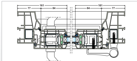
telaio monoblocco - profondità 105 mm
