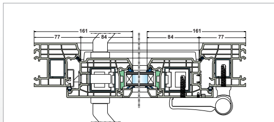
telaio Top 72 - profondità 72 mm
