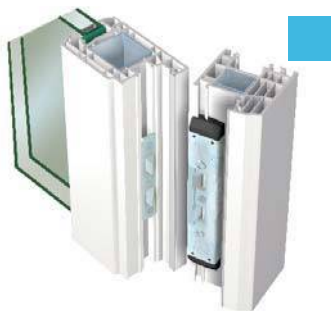
rostri di sicurezza per la protezione contro eventuali tentativi di sfondamento o scasso
