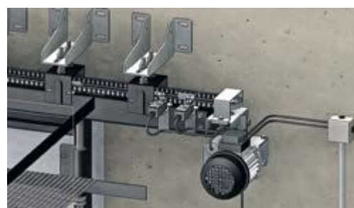
Motorizzazione a catena Motorization with chain Schleppkettenantrieb
