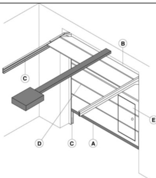
Zone di rischio della porta sezionali da garage (figura 1)
